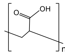
Fig. 2 Chemical structure of PAA.
