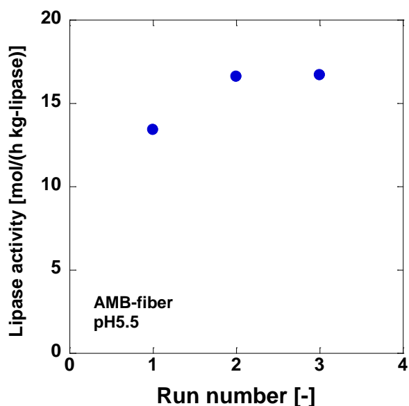
Fig. 5 繰り返し利用による酵素活性の変化
