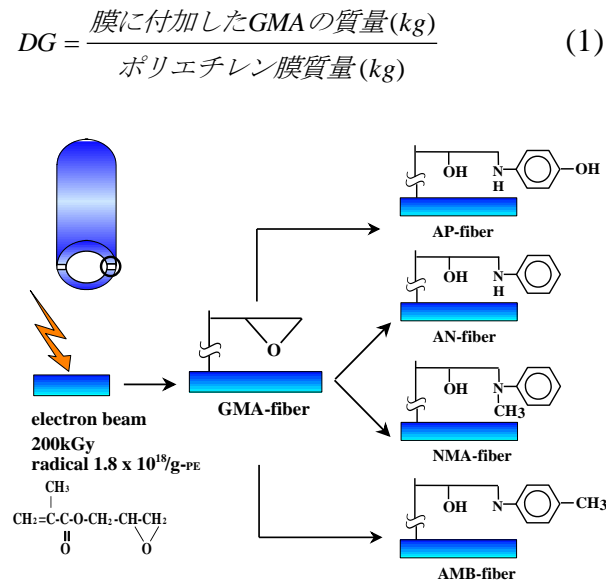
Fig. 2 官能基導入フローチャート
